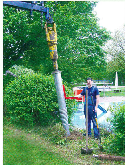
versenktes Schraubgewinde
